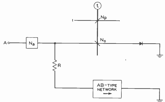
Fig. 19—A pulse timing shunt.
