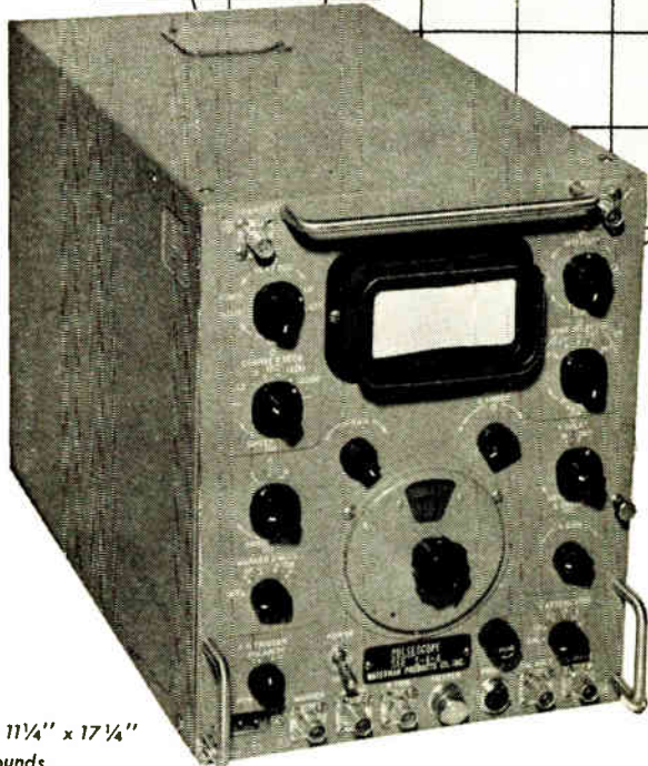
MODEL S-4-A
