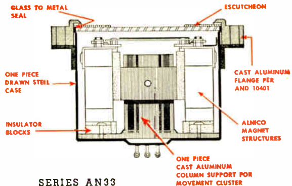
SERIES AN33
