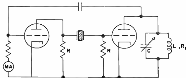
Fig. 9—Heegner circuit.
