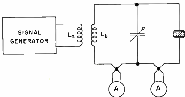
Fig. 11—Crevasse circuit.
