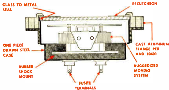
SERIES AN3
