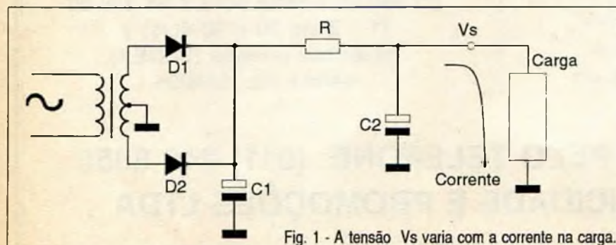
Fig. 1 - A tensão V_s varia com a corrente na carga.
