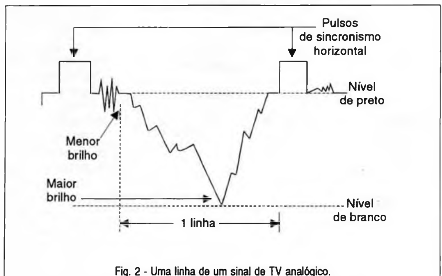
Fig. 2 - Uma linha de um sinal de TV analógico.
