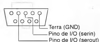
DB-9 (Fêmeas) PC/AT lado da solda
