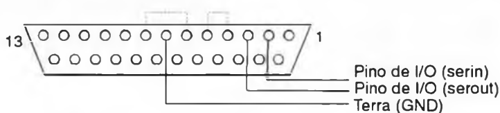
DB-25 (macho) (PC-XT) - lado da solda
