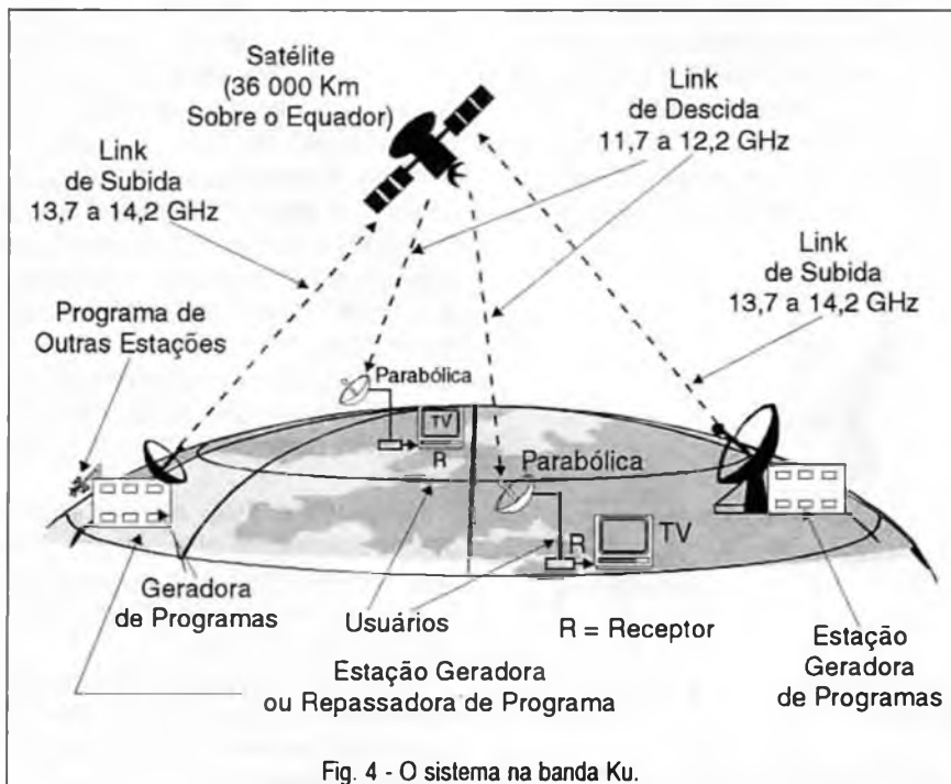
Fig. 4 - O sistema na banda Ku.
